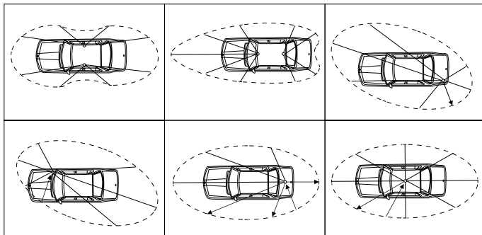
Вид апертуры антенны
